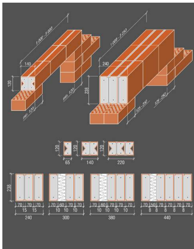
Ukážka použitia keramického prekladu pri preklopení otvoru v rôznej hrúbke muriva
