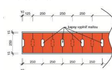
TD 250 PD AKUSTIK
