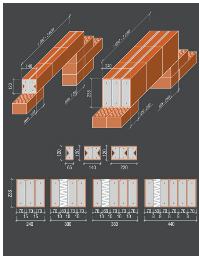
Ukážka použitia keramického prekladu pri preklopení otvoru v rôznej hrúbke muríva
