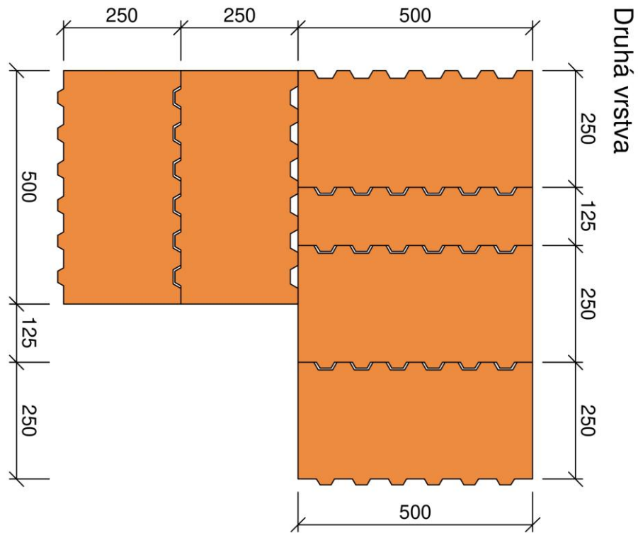
Obrázok 2.1 – Založenie rohu z tehál TermobRIK TD 500 PD
