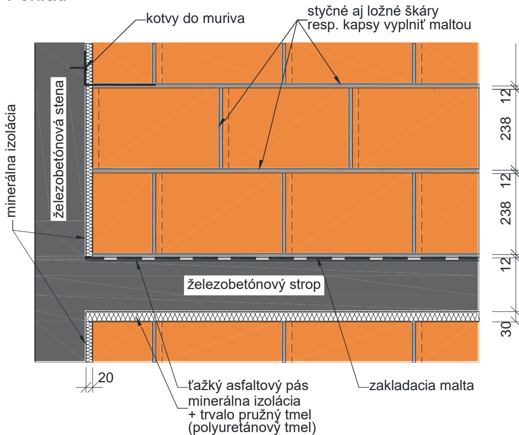
Obrázok 2.15 – Napojenia akustickej deliacej steny na priľahlú železobetónovú konštrukciu – tuhý, resp. pružný spoj v pohľade
