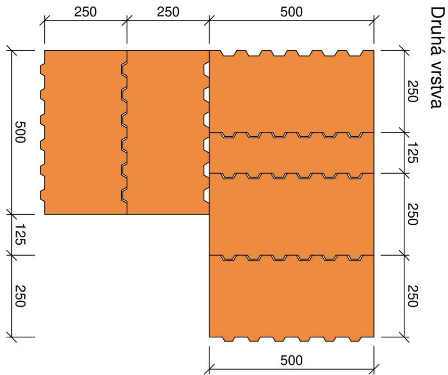
Obrázok 2.1 – Založenie rohu z tehál TermobRIK TD 500 PD
