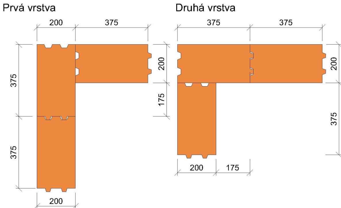
Obrázok 2.6 – Založenie rohu z tehál TermoBRIK TD 200 PD
