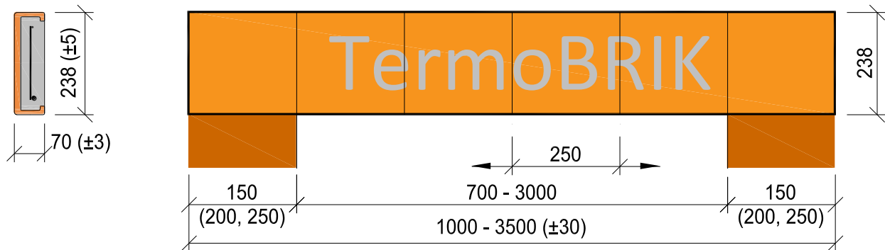
Obrázok 3.8 – Spôsob použitia prekladu KP 23,8
