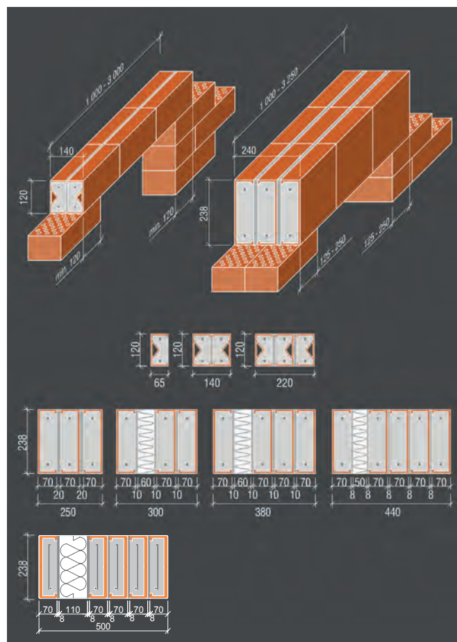
Ukážka použitia keramického prekladu pri preklopení otvoru v rôznej hrúbke muríva
