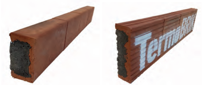
Ukážka použitia keramického prekladu pri preklopení otvoru v rôznej hrúbke muríva
